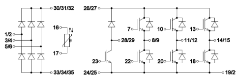
电路示意图
