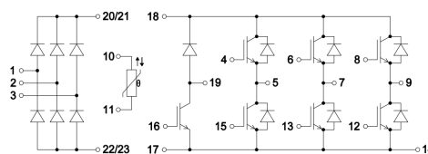
电路示意图
