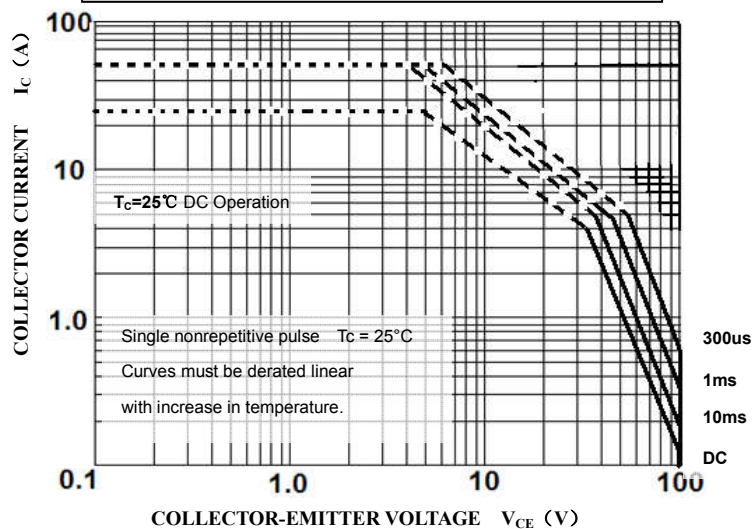
SOA
