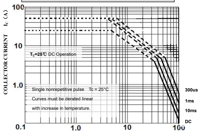
SOA
