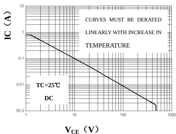
SOA
