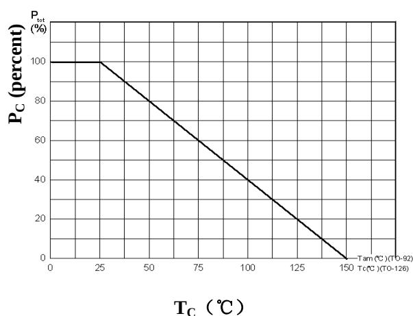
P_C - T_C
