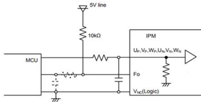
图 11: 推荐的 MCU 输入输出接口电路
