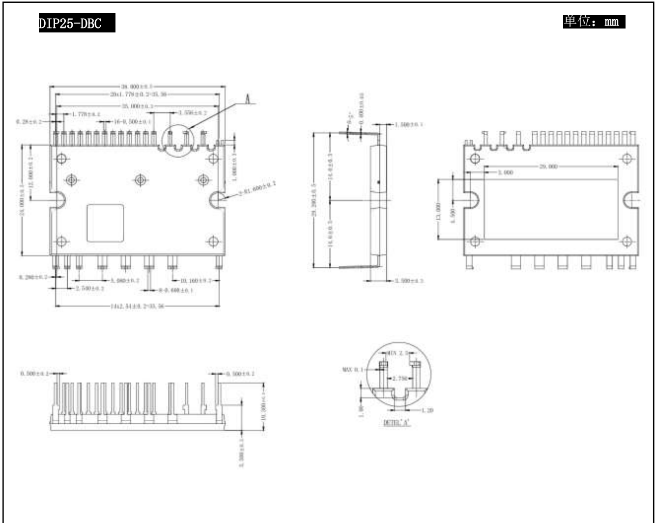
图 14: 封装尺寸示意图
