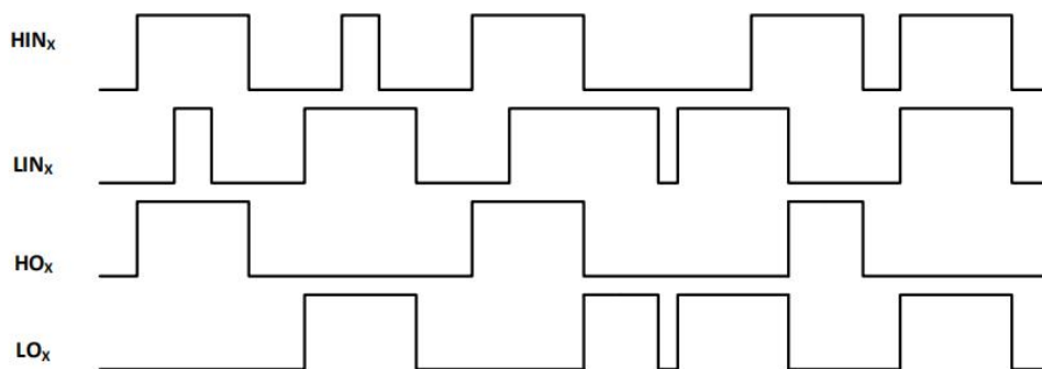
图 10: 直通保护
