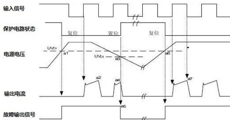
图 11: 欠压保护时序图(低侧)
