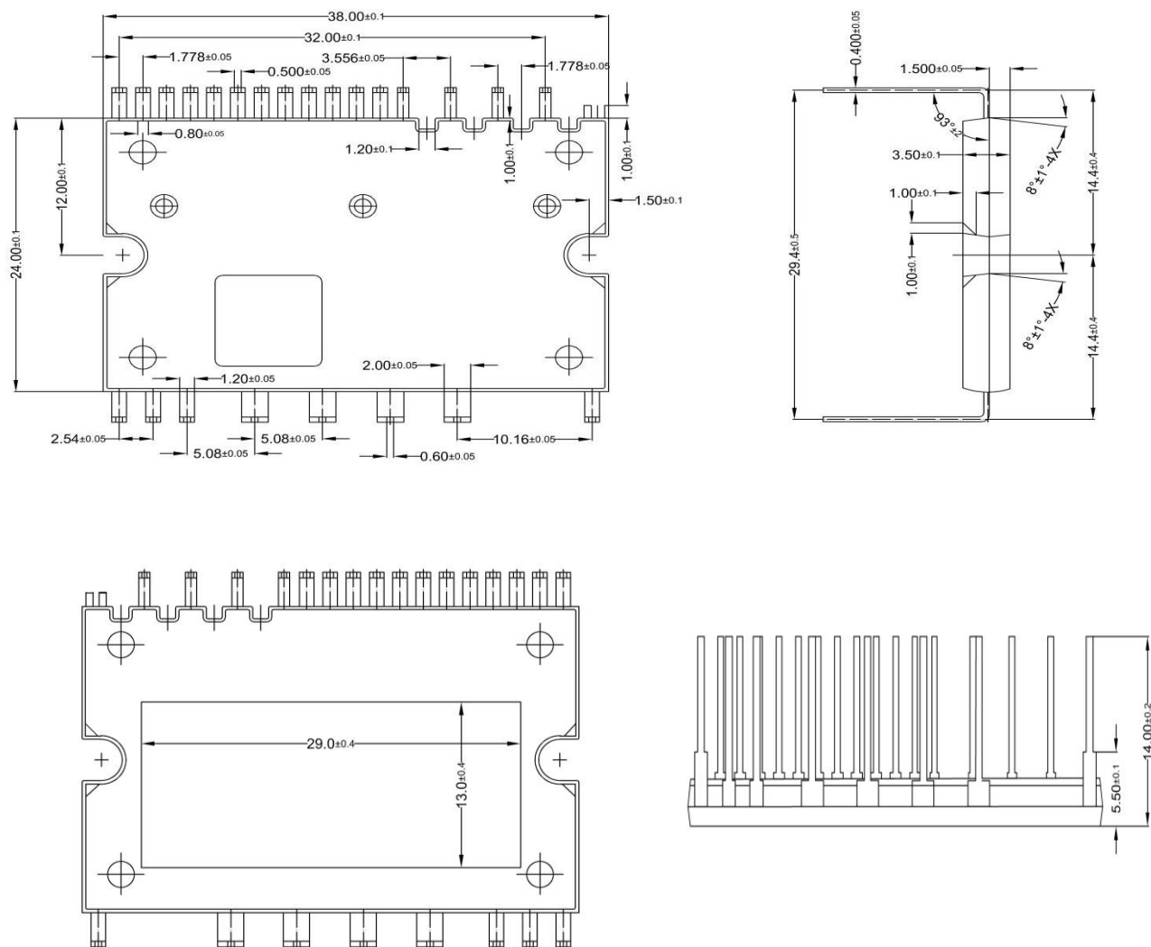
图 17: 封装尺寸示意图
