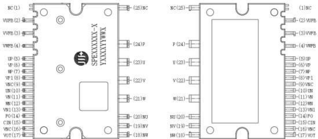
图 2：模块引脚分布示意图
