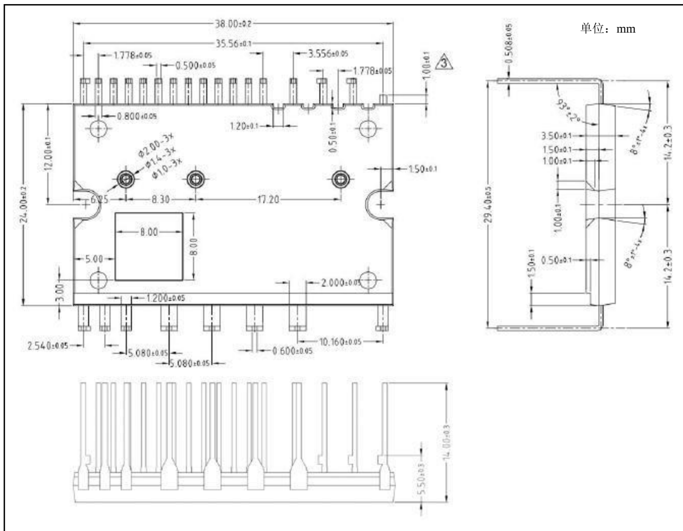
图 17: 封装尺寸示意图
