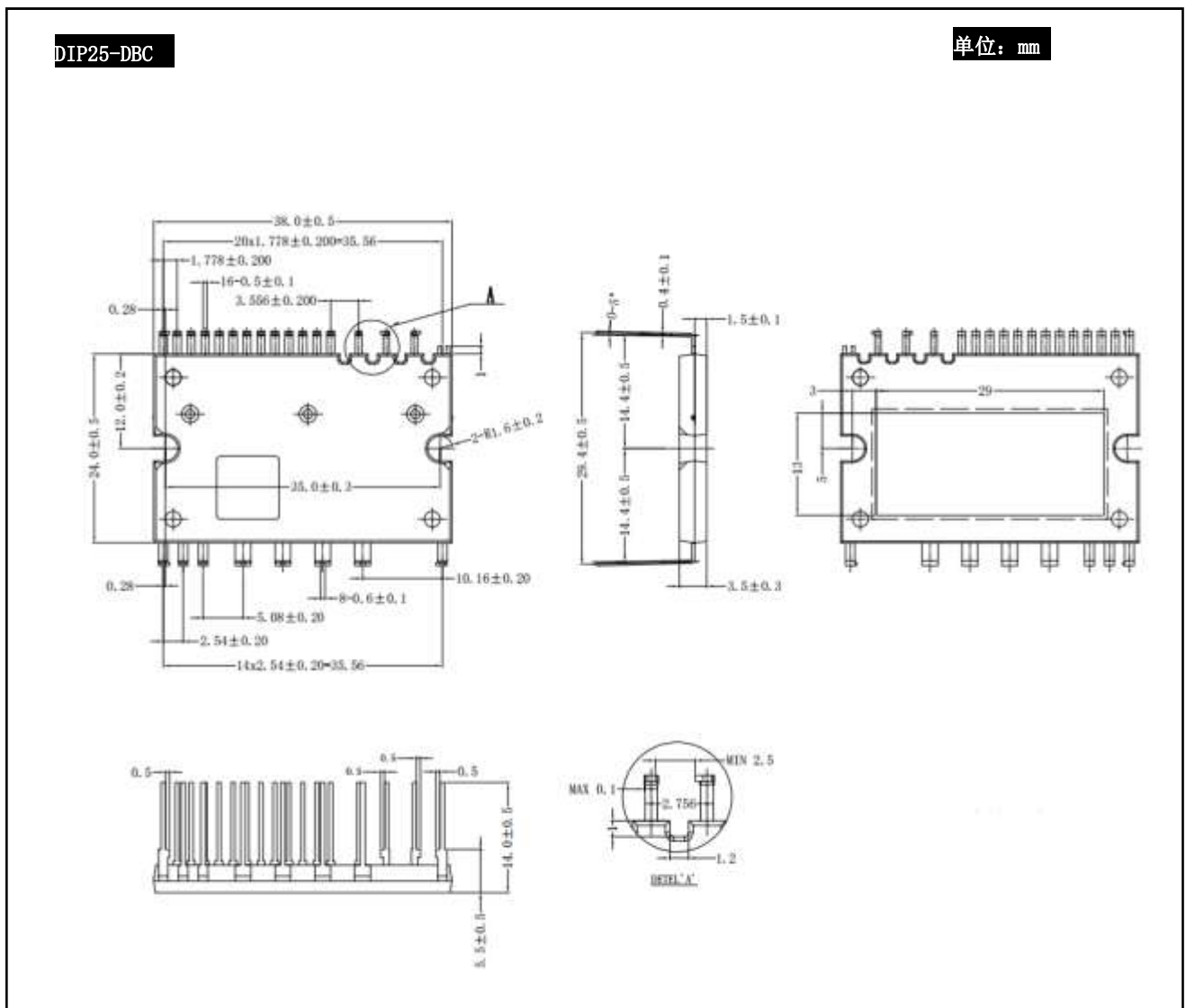
图 14: 封装尺寸示意图
