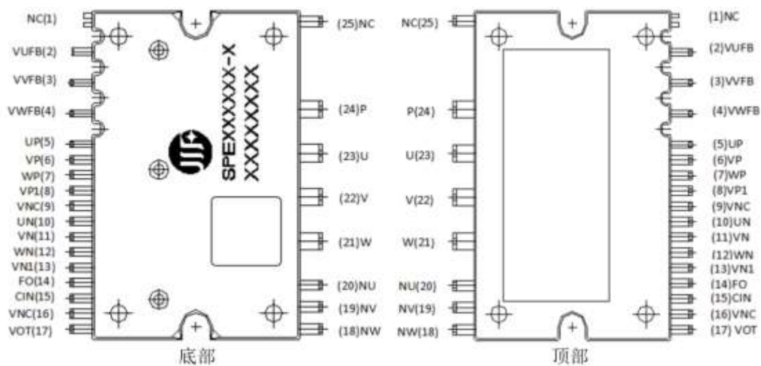
图 2: 模块引脚分布示意图
