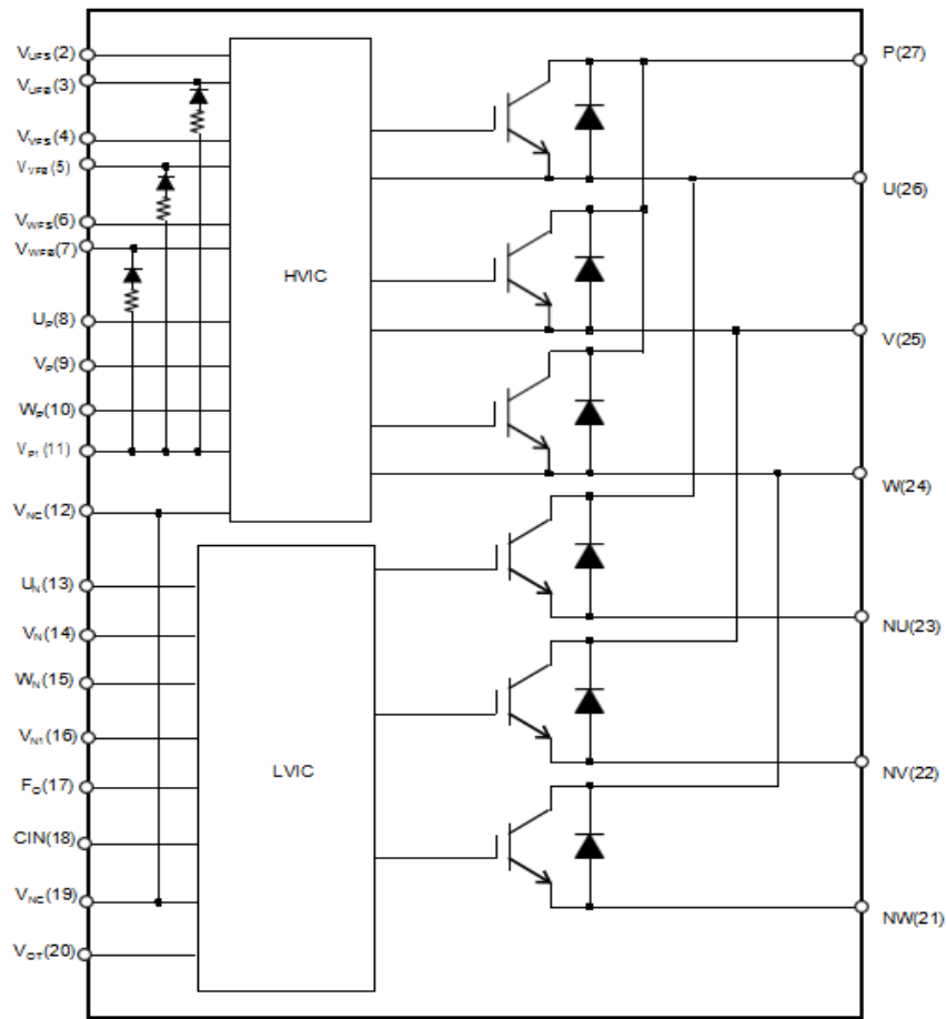
图 1：模块内部电路示意图
