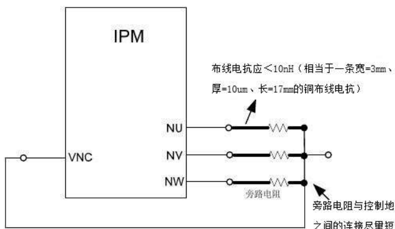
图 14: 旁路电阻接线注意事项
