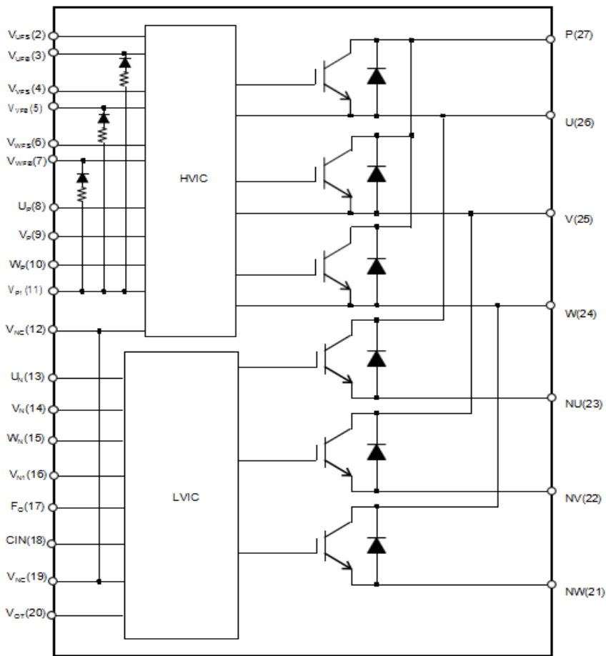
图 1：模块内部电路示意图 Fig 1: Internal circuit
