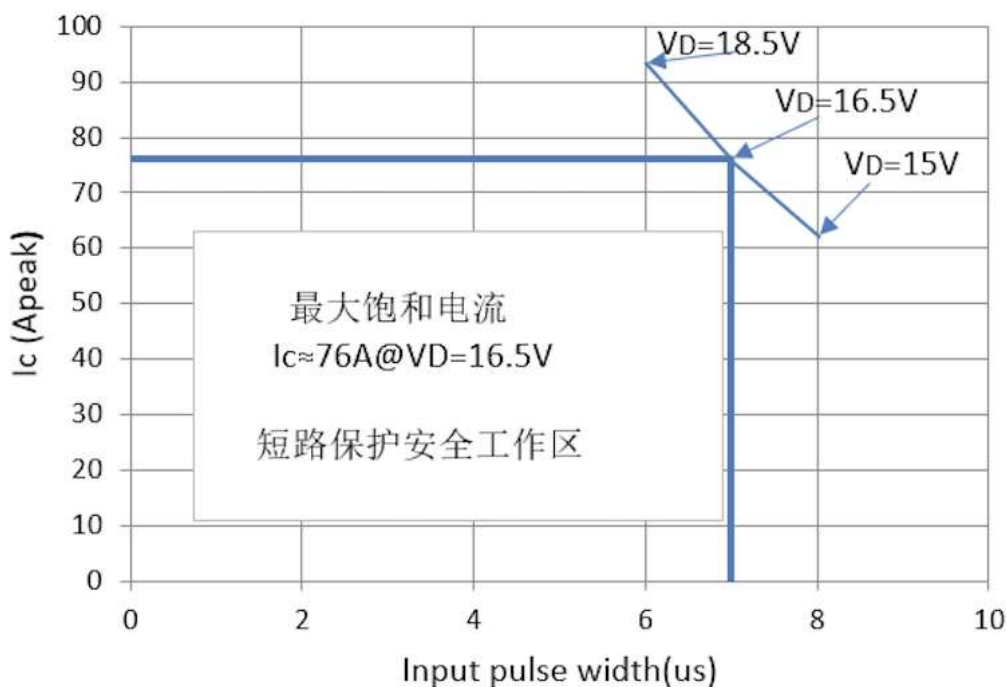
图 15 短路安全工作区曲线
