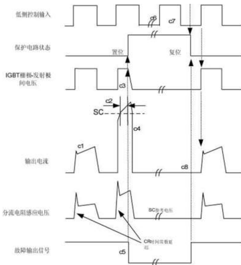
图 12: 短路电流保护时序图 (只适合于低侧)
