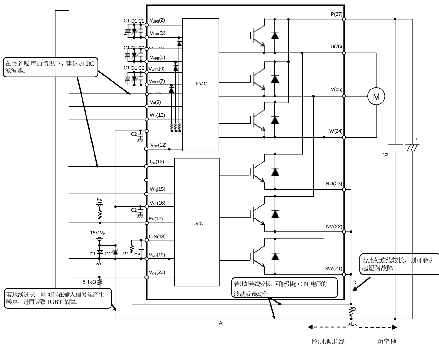
图 16: 典型应用电路
