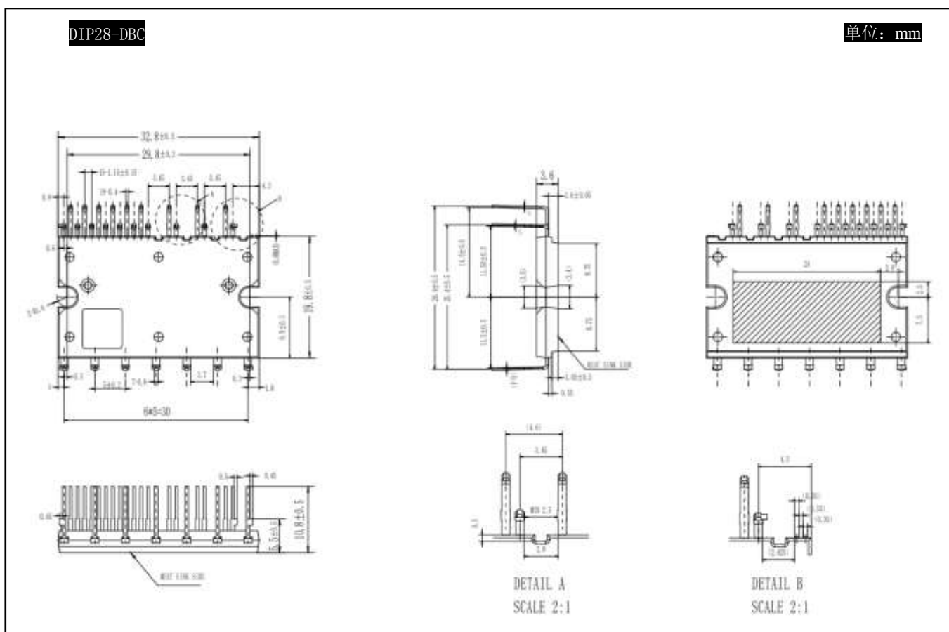
图 18: 封装尺寸示意图
