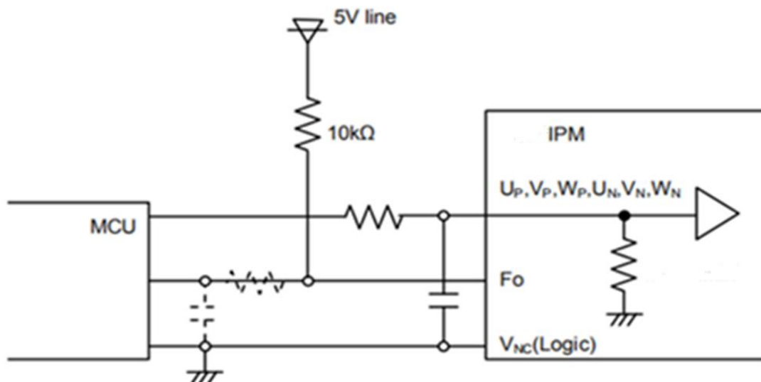
图 11: 推荐的 MCU 输入输出接口电路
