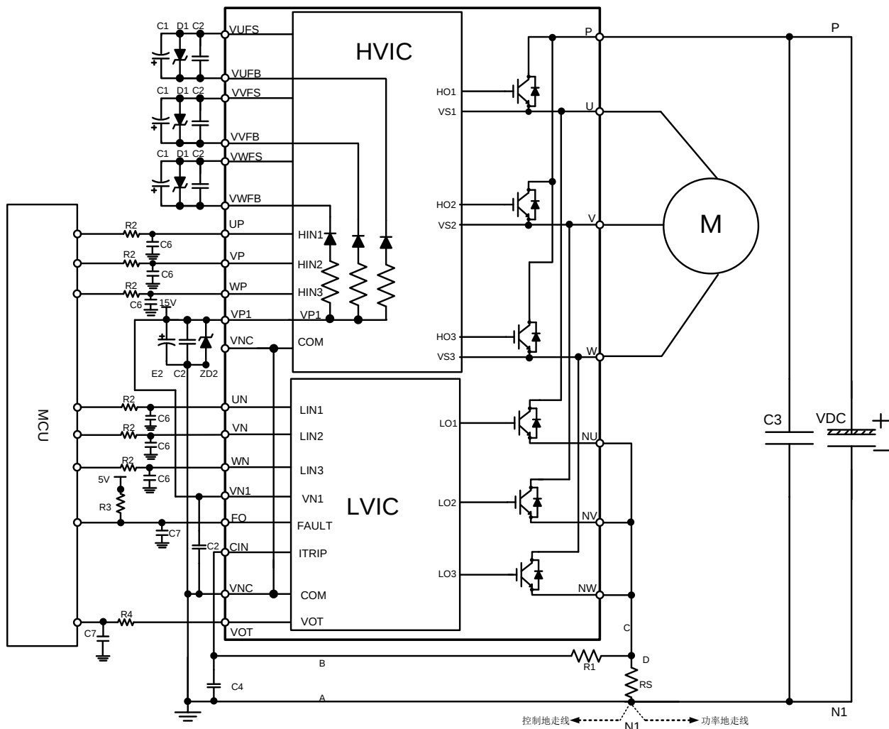
图 13: 典型应用电路
