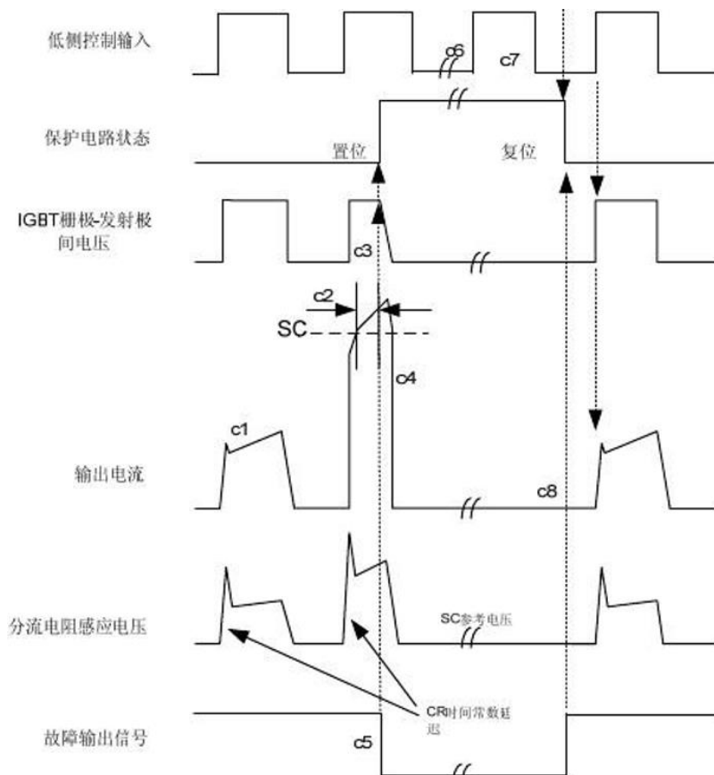
图 10：短路电流保护时序图（只适合于低侧）
