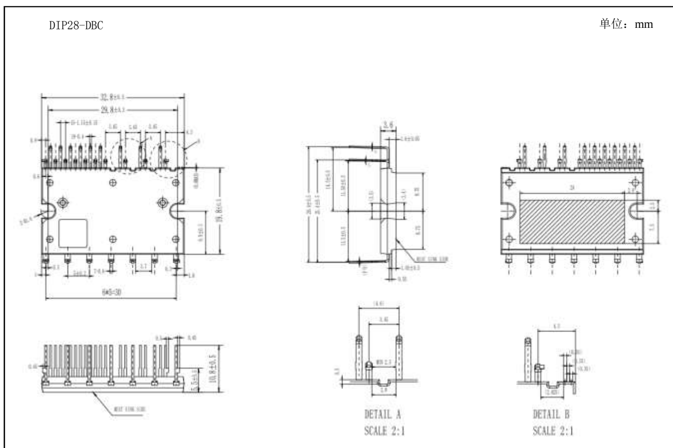
图 14: 封装尺寸示意图
