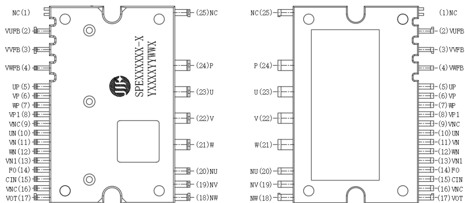
图 2: 模块引脚分布示意图
