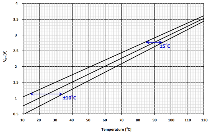
图 6: VOT 输出电压曲线
