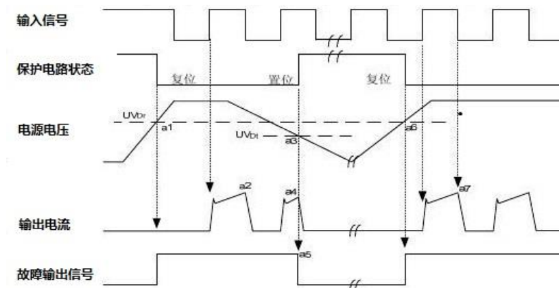
图 8: 欠压保护时序图(低侧)
