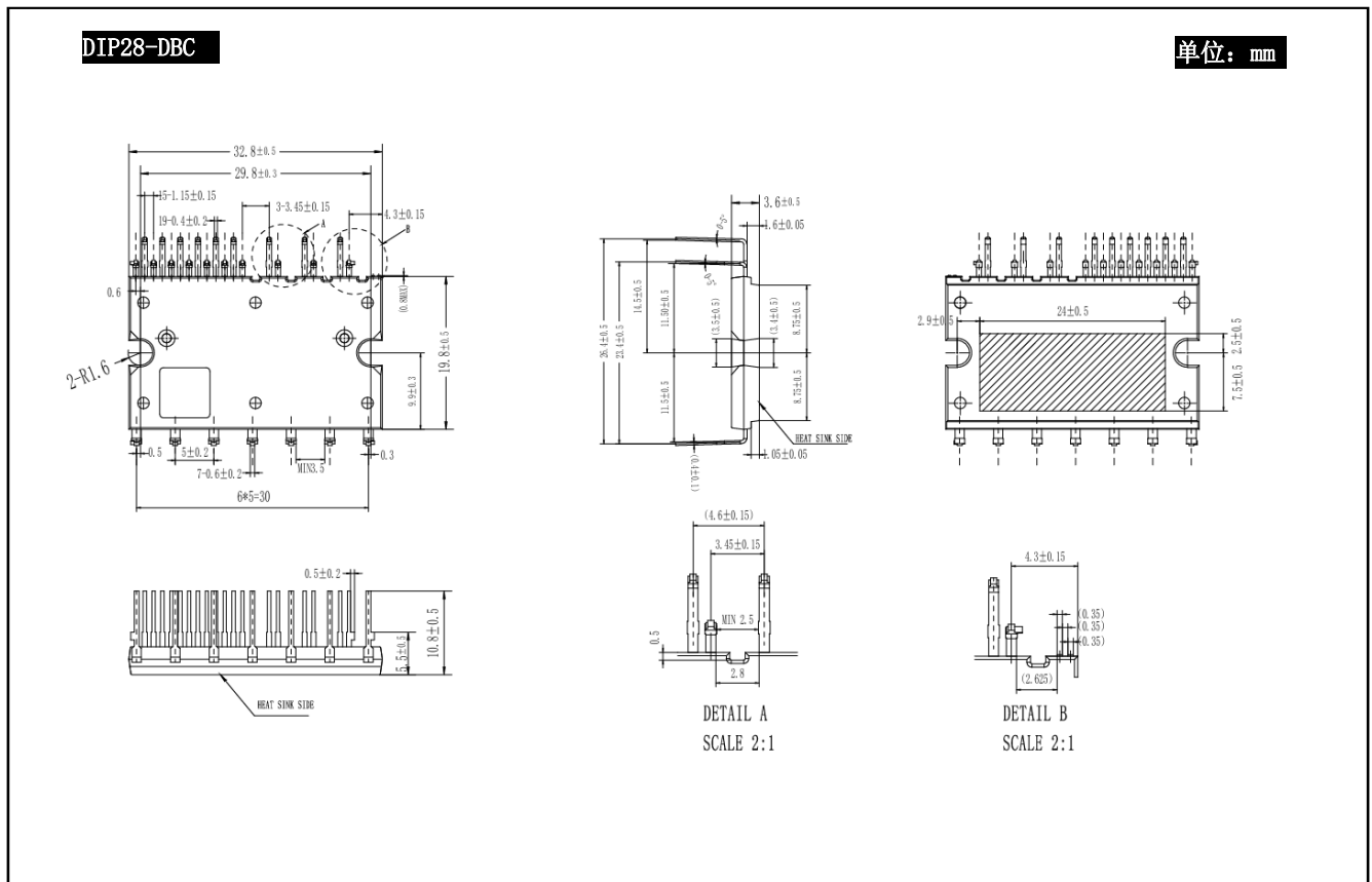
图 14: 封装尺寸示意图
