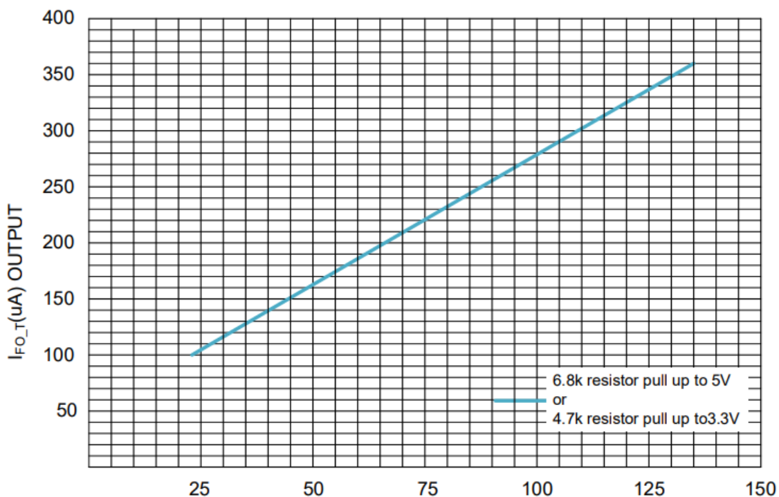
图 5: HVIC 温度检测输出温度—电流曲线
