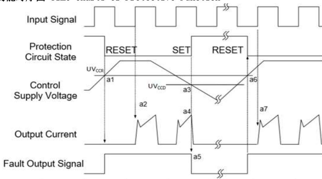
图 6: 欠压保护时序图(低侧)
