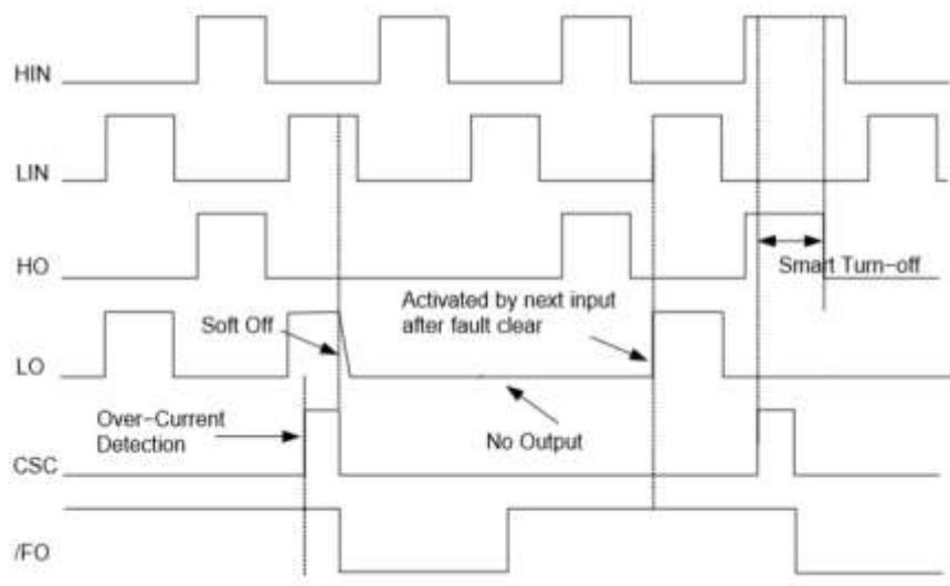
图 7: 过流保护时序
