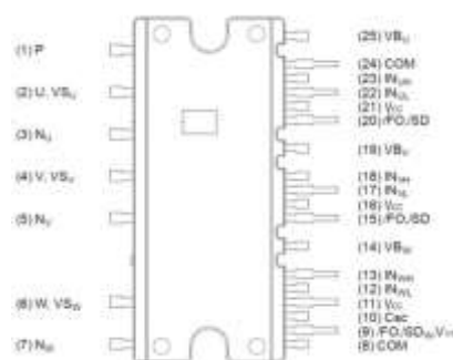
PIN1-PIN25
