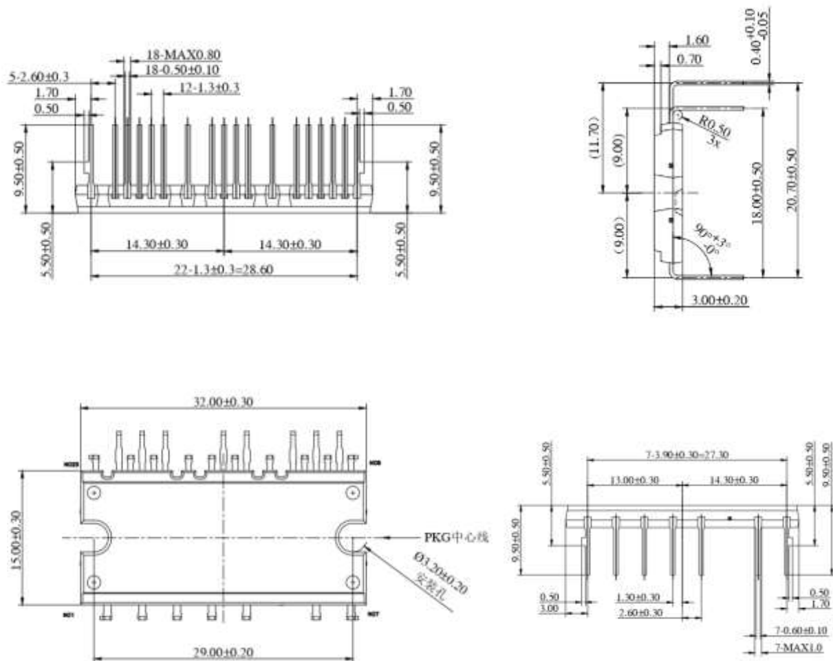
图 11: SPE06S60H-A 封装外形图
