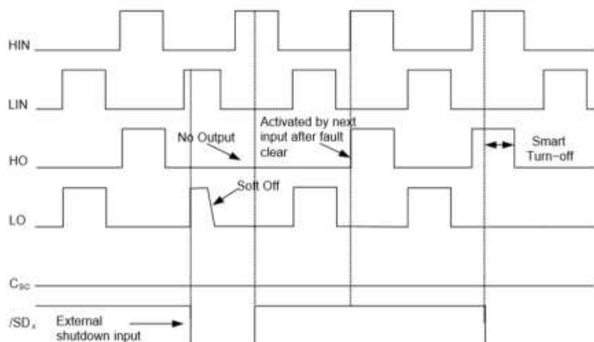
图 8. 外部关断功能时序
