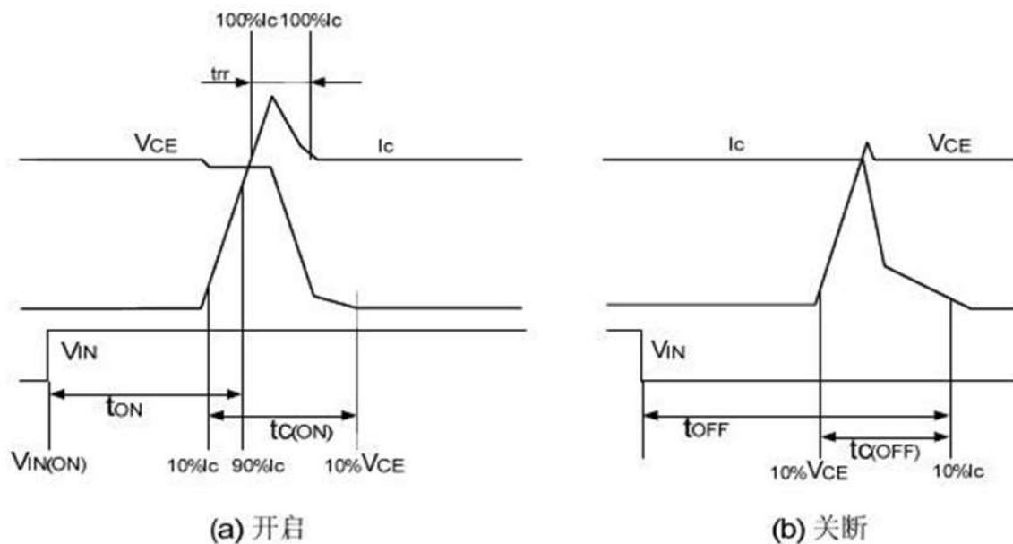
图 5: 开关时间定义
