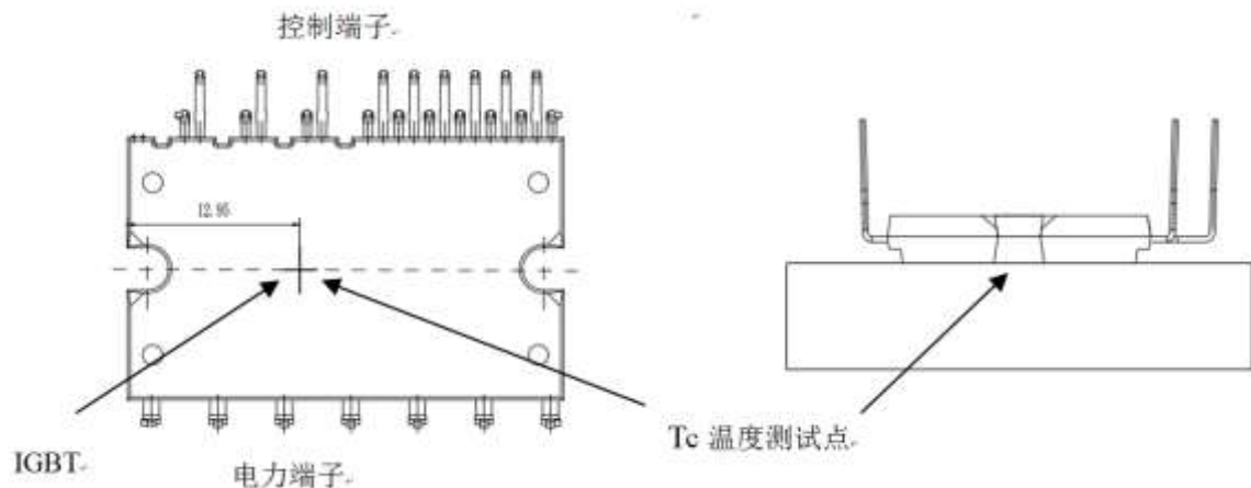
图 4: 壳温 T_c 测试点
