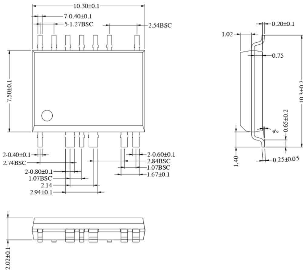
图 11: SPE06S60A-CN 封装外形图
