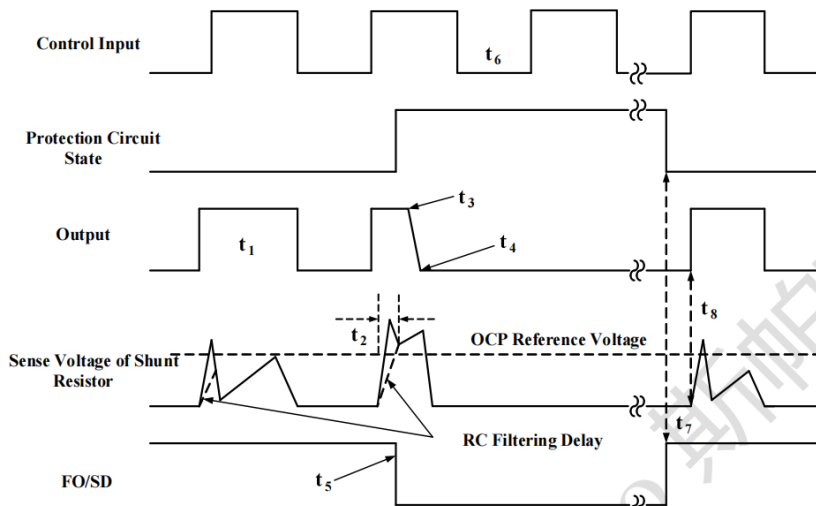
图 8：短路保护时序图
