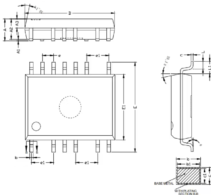
图 12: SPE06S60A-CN 封装外形图
