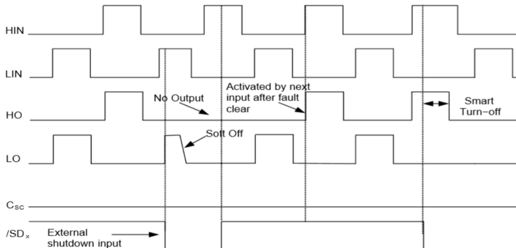
图 9. 外部关断功能时序
