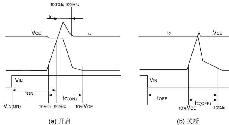
图 4: 开关时间定义
