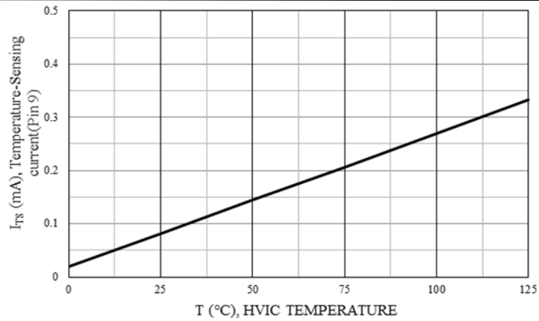
图 5.1: IC 温度输出的电流-温度曲线
