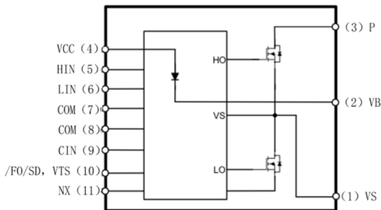
图 1: 模块内部电路示意图
