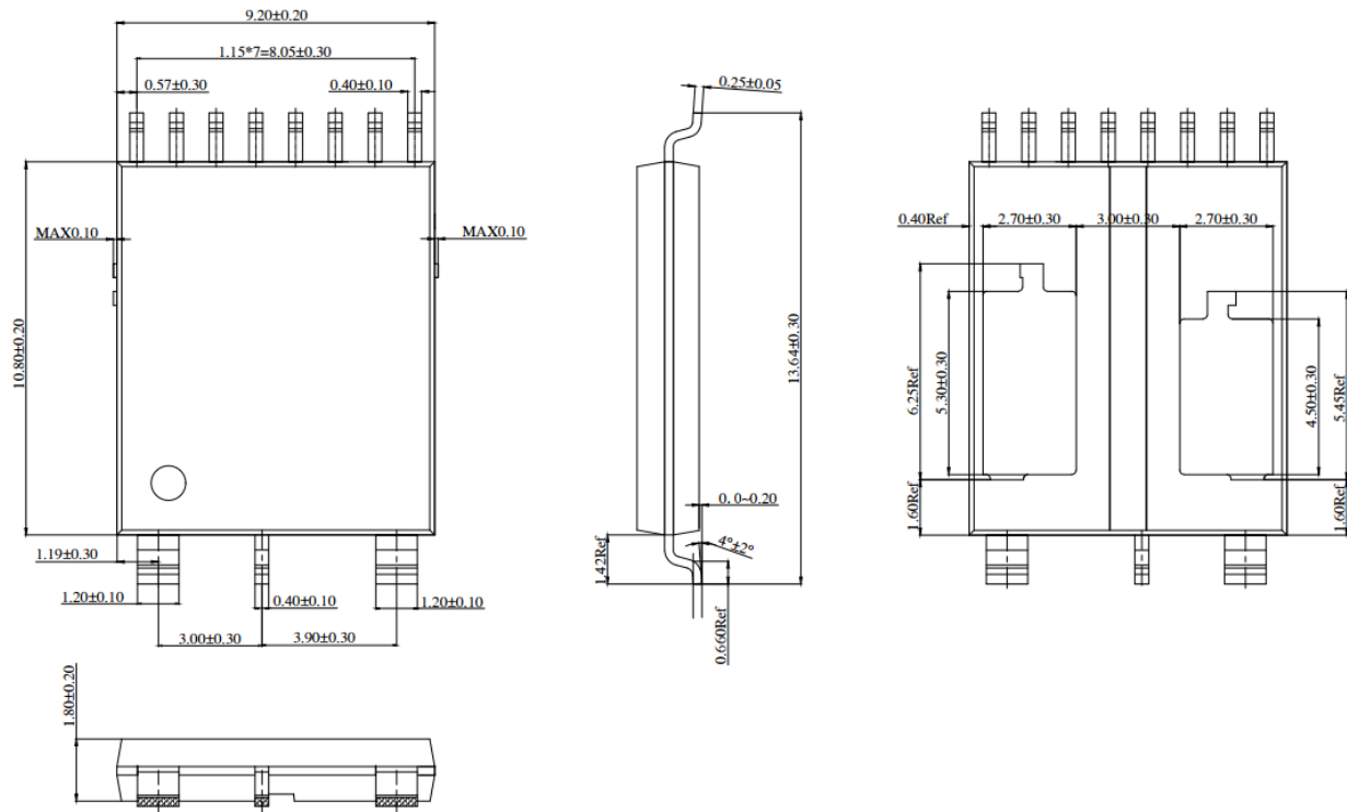
图 12: SPE04M60B-CH 封装外形图
