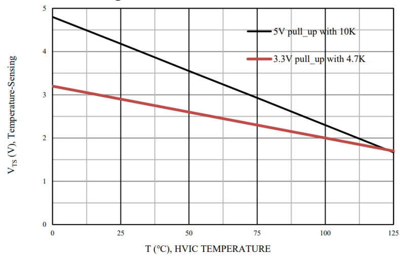
图 5.2: HVIC 温度检测输出温度-电压曲线
