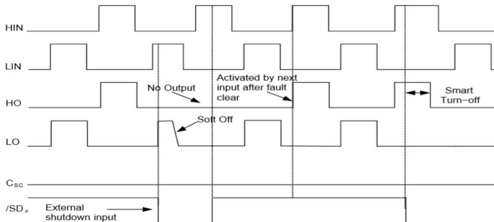
图 9. 外部关断功能时序
