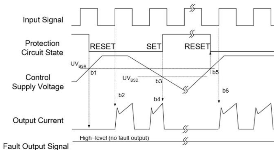
图 8：短路保护时序图
