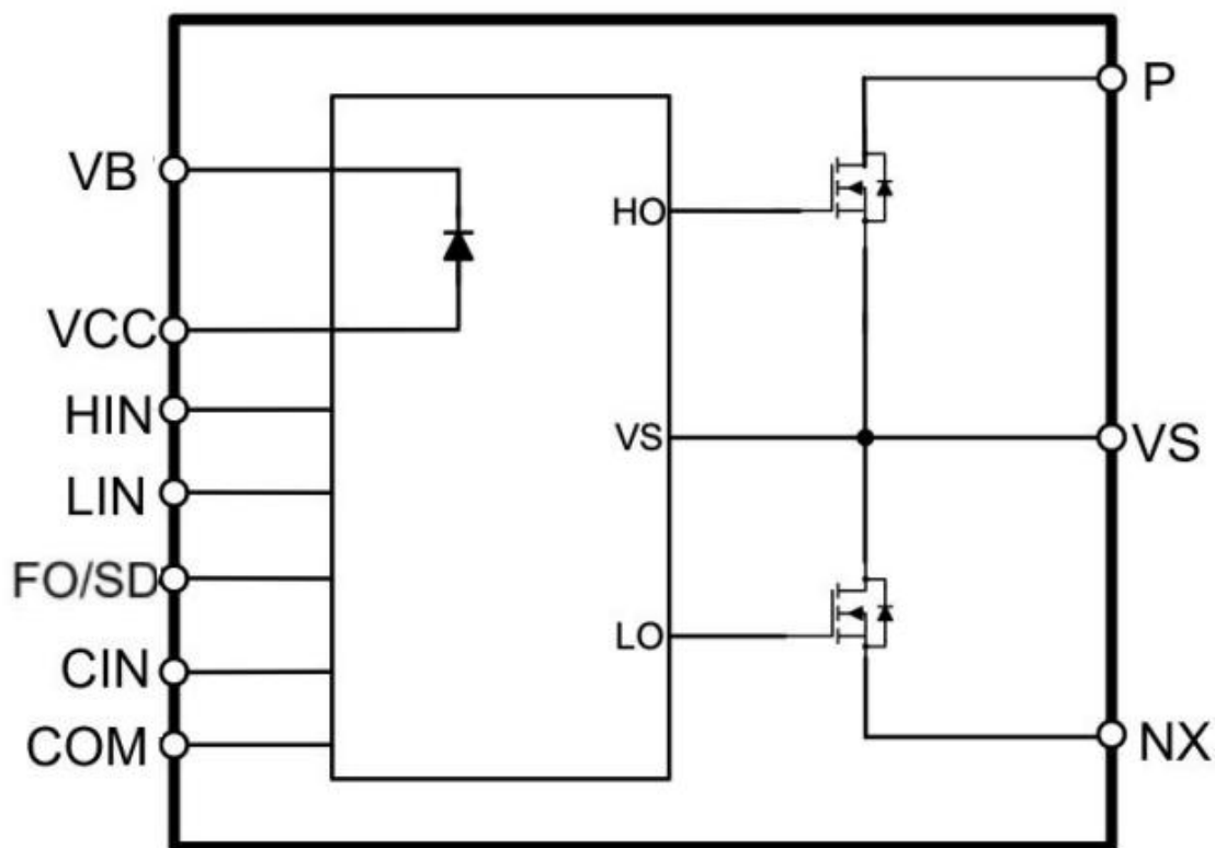
图 1：模块内部电路示意图
