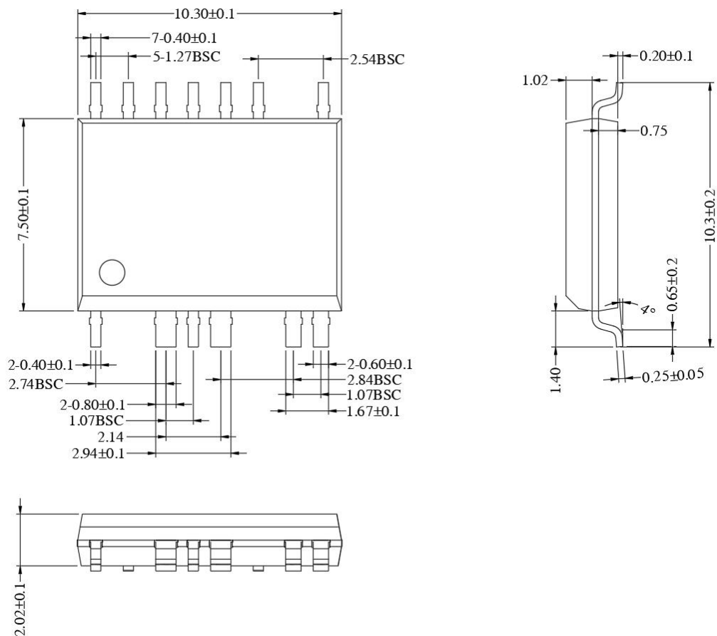
图 11: SPE04M60A-CN 封装外形图
