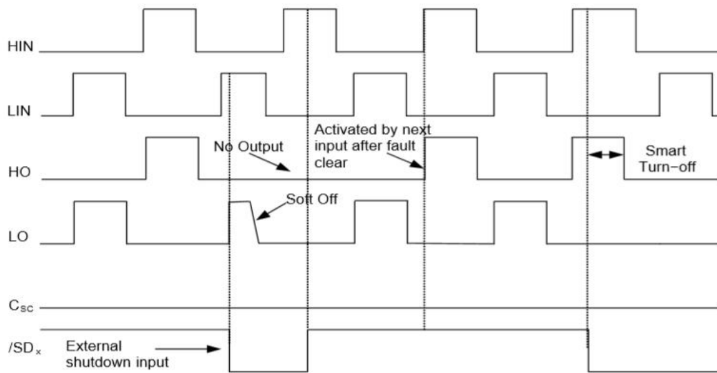
图 9. 外部关断功能时序
