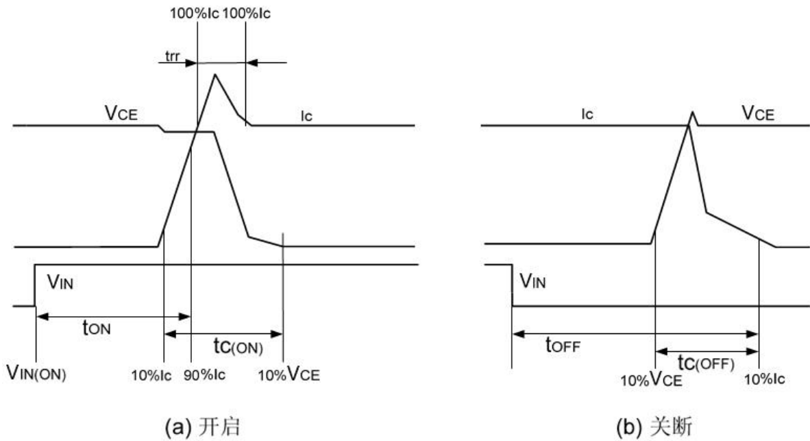
图 5：开关时间定义
