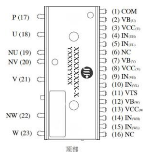
PIN1-PIN23
