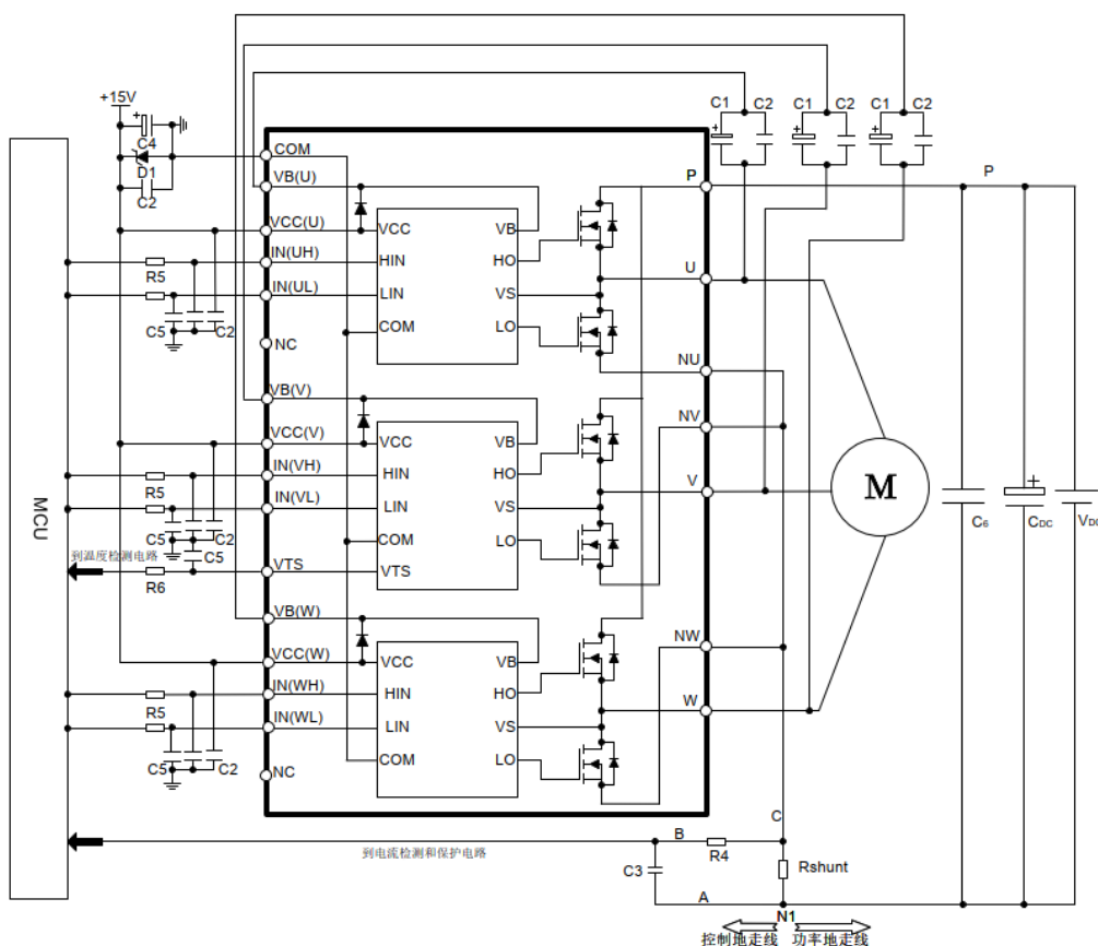
图 10: 典型应用电路图
