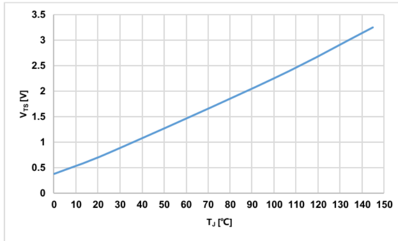
图 5: HVIC 温度检测输出温度—电压曲线
