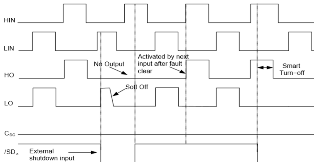
图 9. 外部关断功能时序
