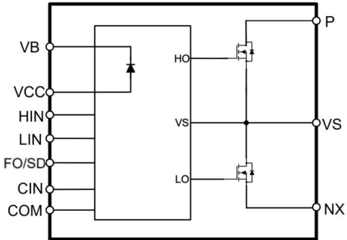
模块分布示意图 Module distribution diagram
