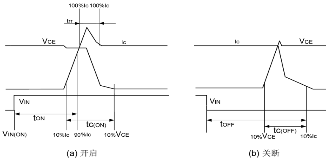
图 4: 开关时间定义
