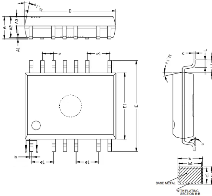
图 12: SPE03M60A-CN 封装外形图
