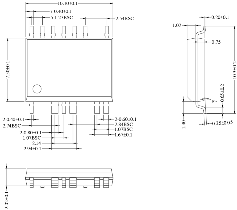
图 11: SPE03M60A-CN 封装外形图
