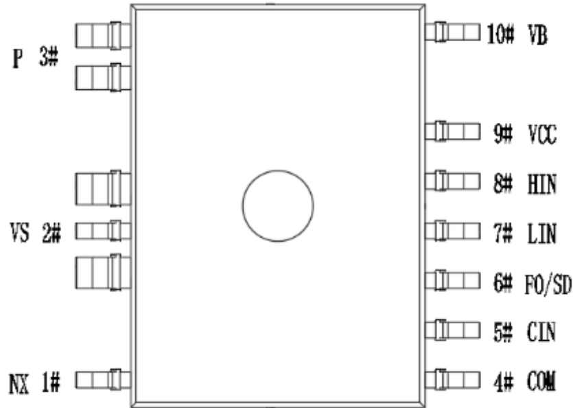
图 2.2: 背面引脚分布示意图
