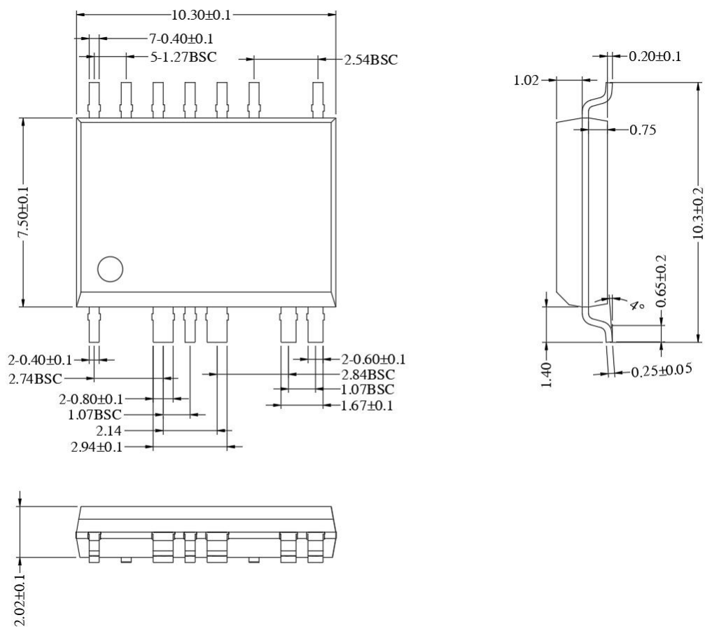
图 12: SPE03M60A-CN 封装外形图
