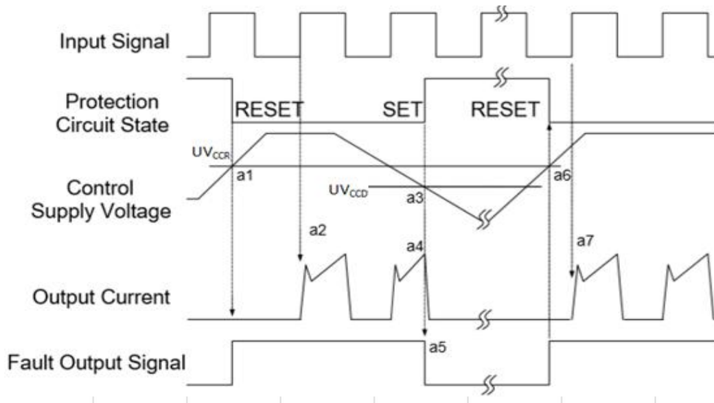
图 8：欠压保护时序图(低侧)
