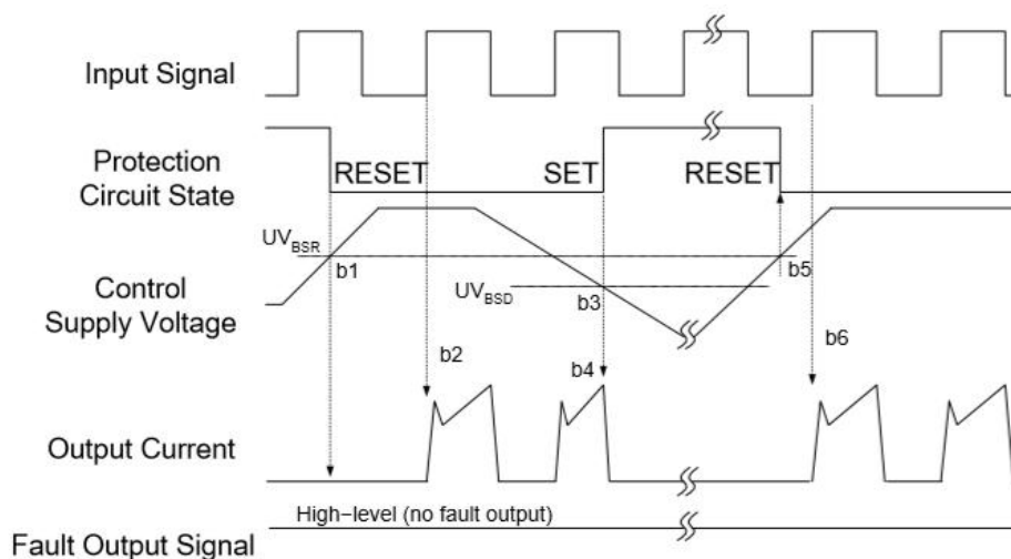
图 9：短路保护时序图
