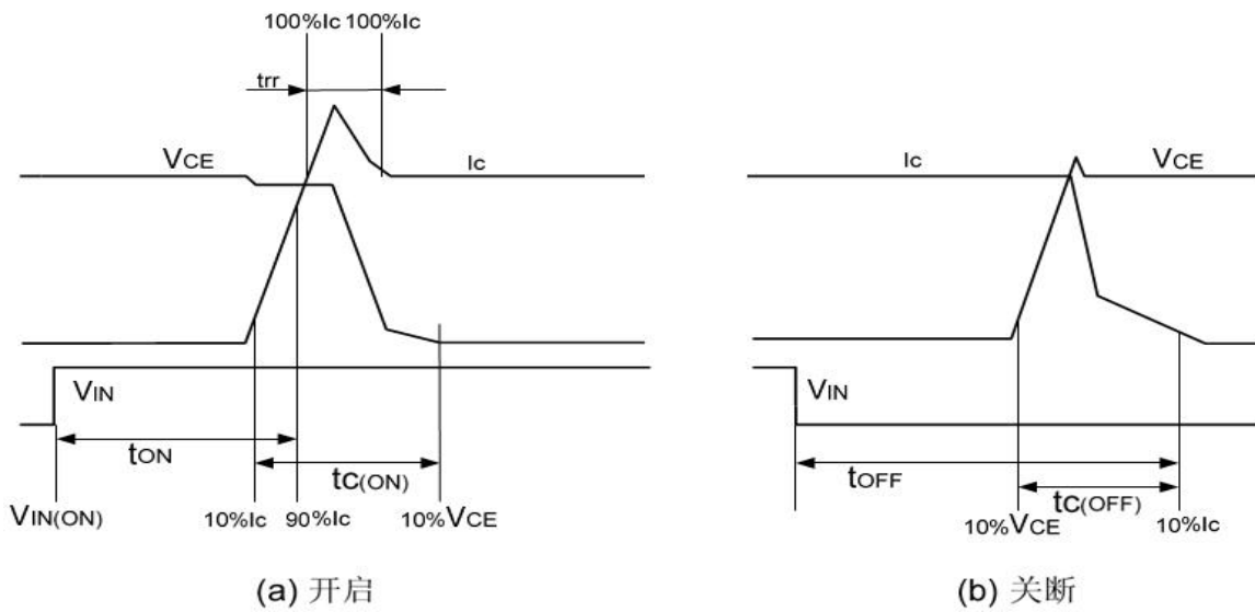
图 5: 开关时间定义
