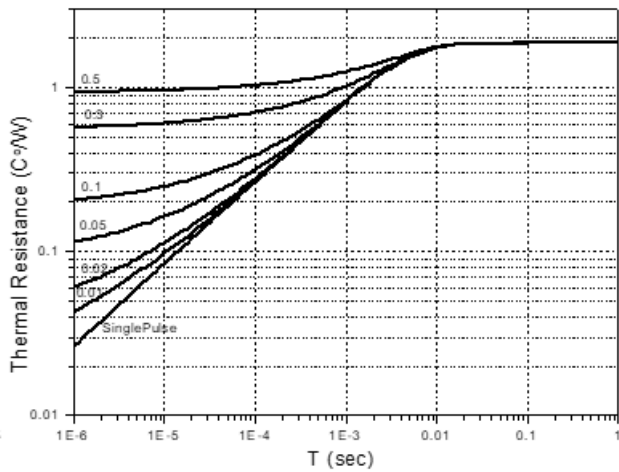
Transient Thermal Impedance (DPAK)
