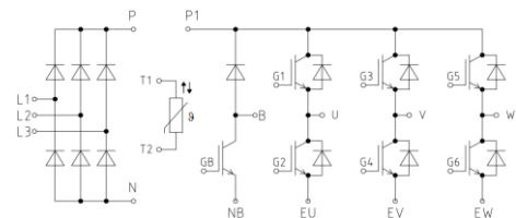
电路示意图
