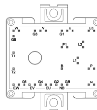
引脚示意图
