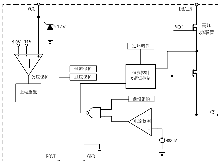
图 3 JH3221B 内部框图
