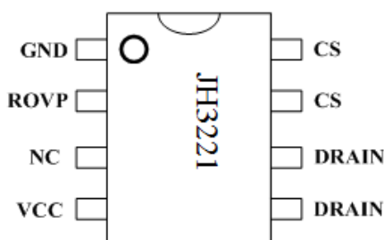
图 2 管脚封装图
