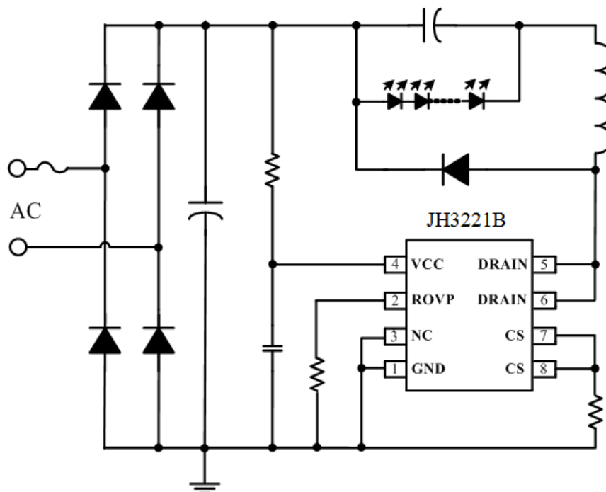
图 1 JH3221B 典型应用图
