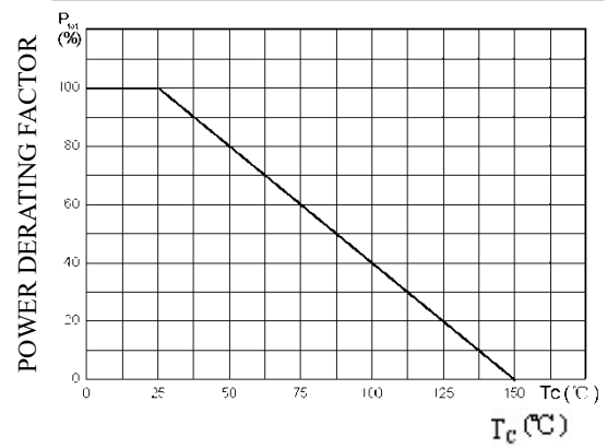
P_C - T_C
