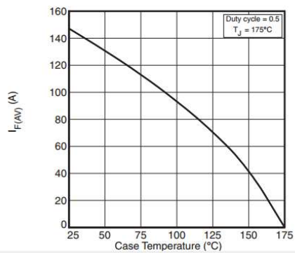
I_F vs T_C
