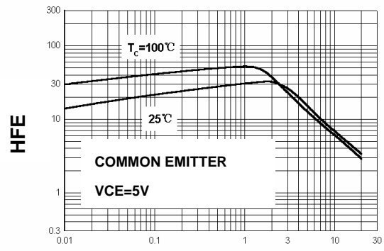
HFE - IC
