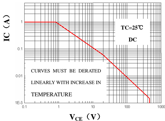
SOA
