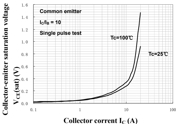
V_{CE(sat)} - I_C
