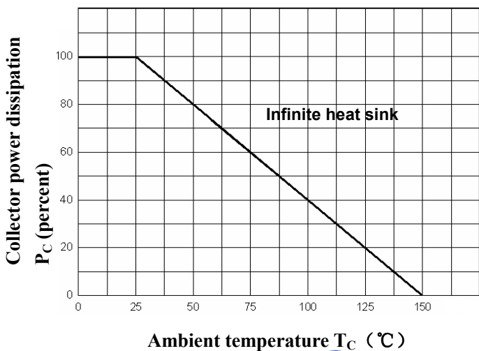
P_C - T_C
